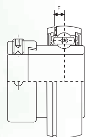
SA 2S anello esterno sferico, con sede per seigeer outer spherical ring, with groove for snap ring
